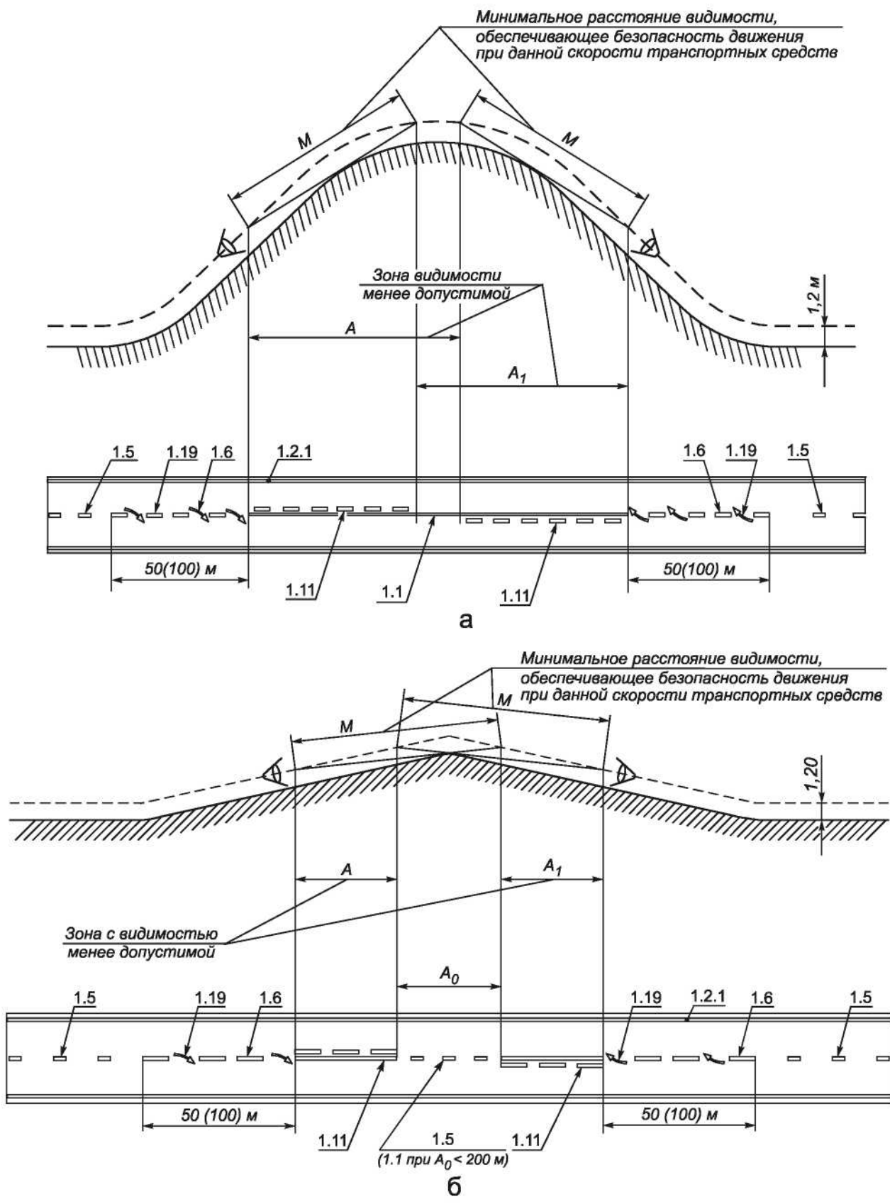
Рисунок В.6 - Примеры нанесения разметки на участках дорог с небезопасной видимостью, где зоны видимости встречного автомобиля: а - перекрываются; б - не перекрываются
