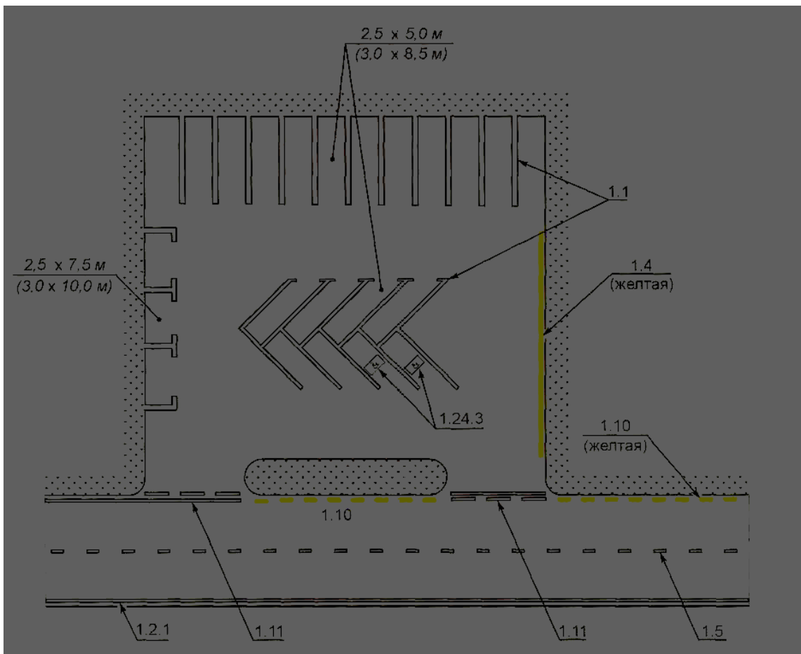
Рисунок В. 13 - Пример нанесения разметки на площадках, предназначенных для стоянки транспортных средств
