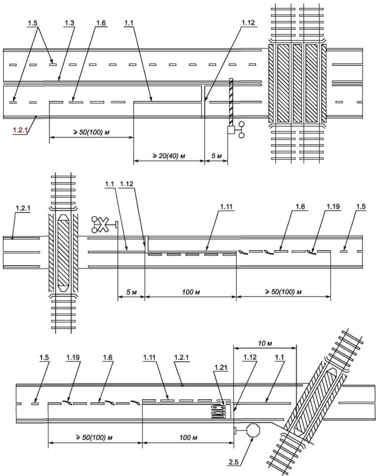
Рисунок В. 17 - Примеры разметки участка дороги на подъезде к железнодорожному перезду
