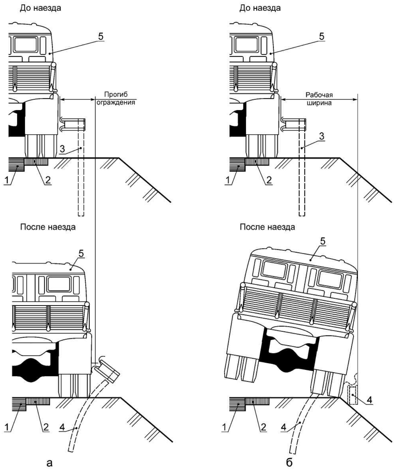
Рисунок В.25 - Динамический прогиб ограждения
